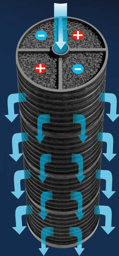
Représentation simplifiée de la technique à quadrupôle
